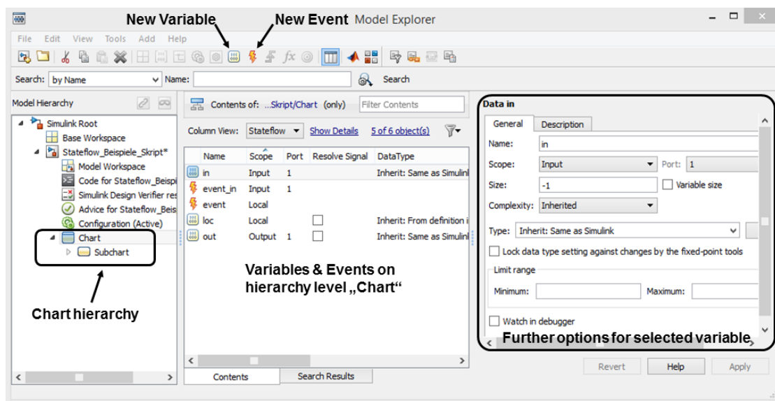
Abbildung 54: Stateflow Model-Explorer
