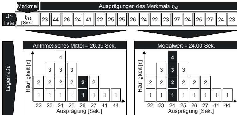
Abbildung 10-4: Grundbegriffe der deskriptiven Statistik und Einführung der wesentlichen Maßzahlen von Häufigkeitsverteilungen (in Anlehnung an VOGEL (1991), ECKSTEIN (2012))
