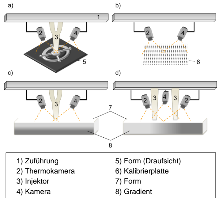
Abbildung 1: Schematischer Aufbau der Gießanlage mit Thermo-Stereo-Kamerasystem a) in der Gießanlage, b) für die Kalibrierung, c) Y-Variante mit horizontalem und d) II-Variante mit vertikalem Gradienten
